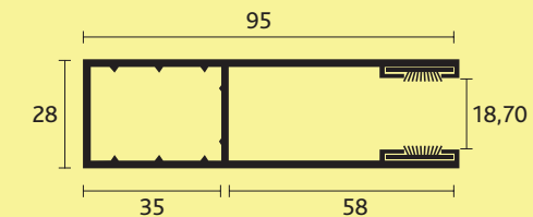
Doorsnede zijgeleider RE-1500 en RE-2000.
