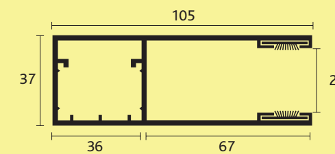
Doorsnede zijgeleider RE-78, RE-87 RE-3000 en RE-M10.
