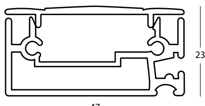
Doorsnede profiel van vaste hordeur.
